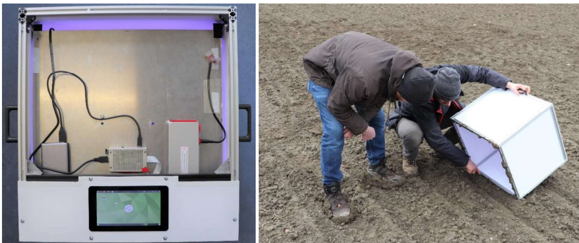
Abbildung 26 Mobile Fotobox zur Datensammlung für die automatische Zielerkennung. Links: Fotobox (Version 1) bestehend aus RaspberryPi, Display und Batterien, sowie LEDs zur Beleuchtung der Feldfläche und Kamera auf der Unterseite. Rechts: Praxiseinsatz der Fotobox V1.
