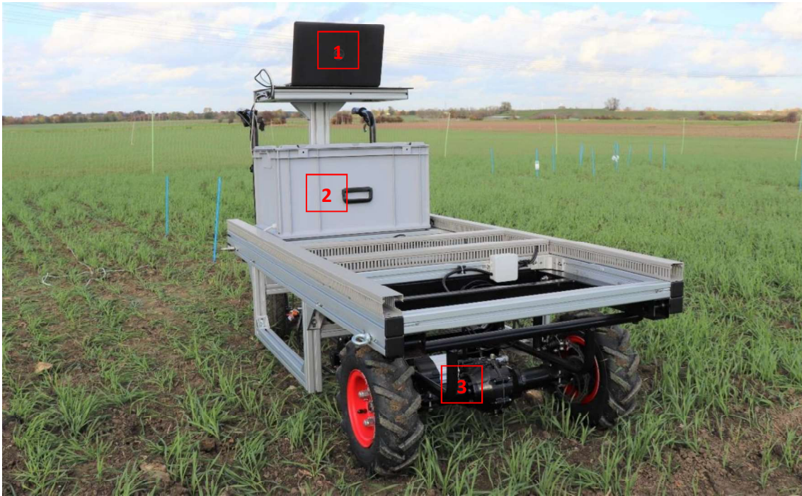
Abbildung 20 Erste Feldbegehung mit dem Trägerfahrzeug inklusive Laserapplikator. Das Trägerfahrzeug beinhaltet u. a.: Eine Steuereinheit für den Laserapplikator (1), eine sichere Einhausung von Steuerungselektronik und Energieversorgung (2) sowie ein 2D-Achssystem (3).
