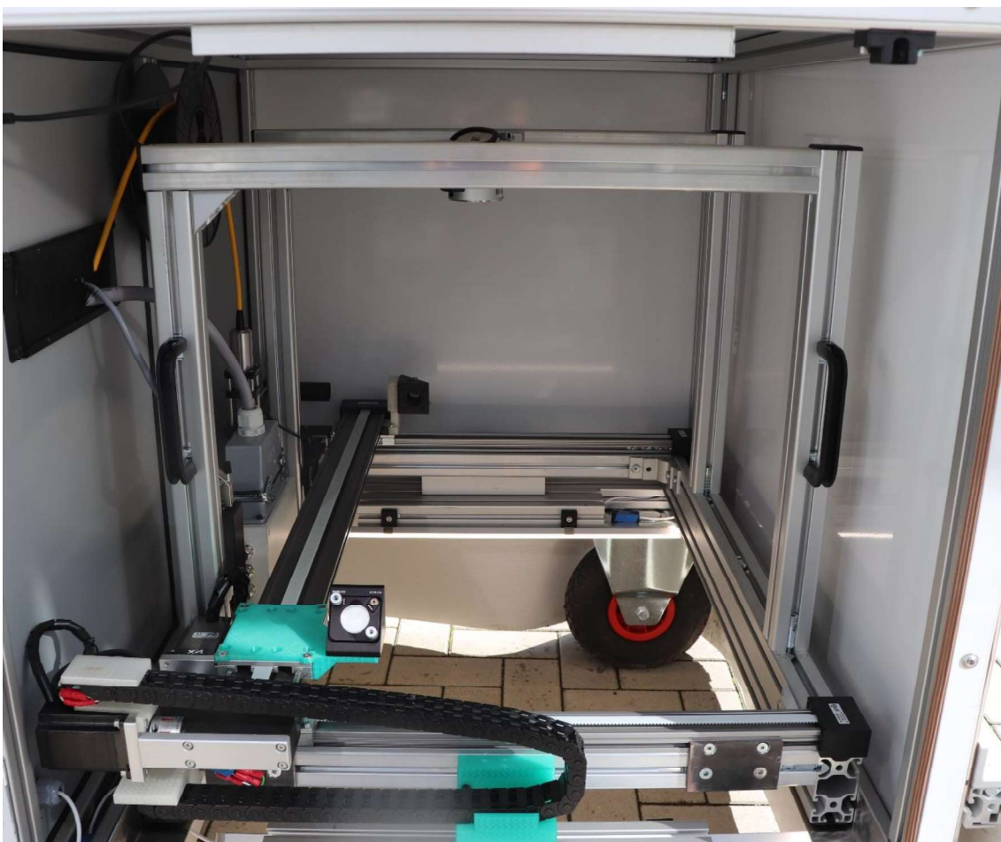
Abbildung 23 Arbeitsraum des Laserapplikators bestehend aus Achssystem, Strahlumlenkung mittels Spiegeln, LED-Beleuchtung sowie einer LIDAR-RGB Kamera.
